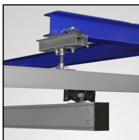
Justerbar upphängningskombination förenklar monteringen
