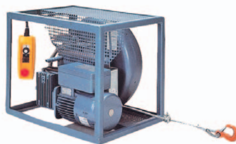
PMH Tirak med inbyggd linhaspel.
