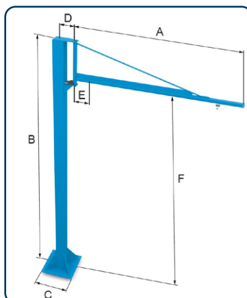
Måttskiss pelarsvängkran FREJ
