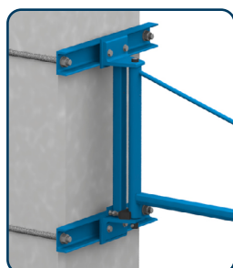
Anpassningsbart väggfäste för olika pelardimensioner**
