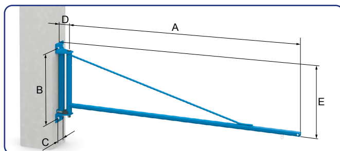
Måttskiss väggsvängkran Frej
