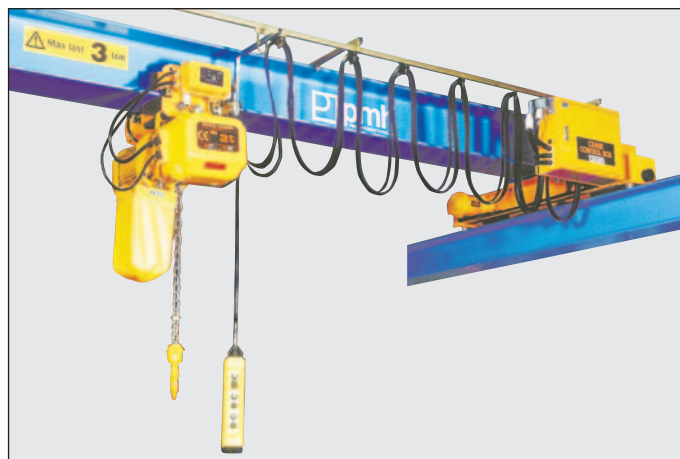
PMH Kabelskena för ström- och manövertillförsel av telfer i traverskran.
