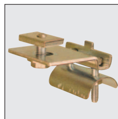
Ändklämma för plattkabel (Max 5 ledare) Typ 1335E
