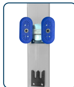
Sugfotshållare
