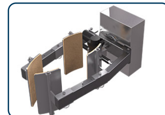
Gripverktyg C
