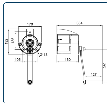
Måttskiss WE 300 &amp; WE 500
