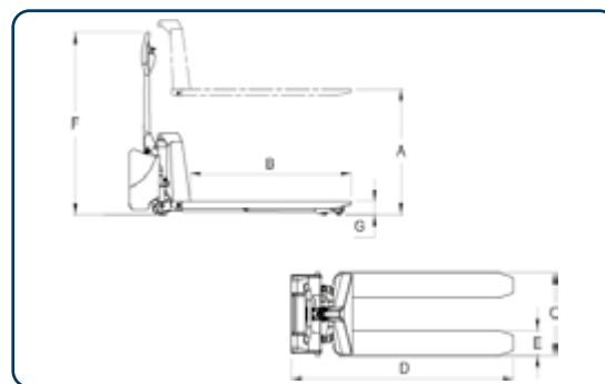
Måttskiss Höglyftare HL
