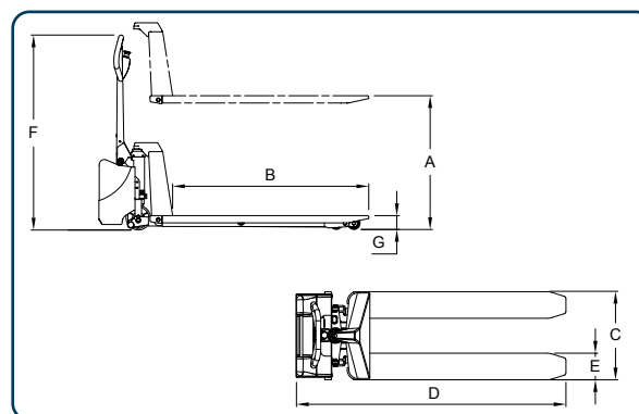
Måttskiss Rostfri gaffellyftvagn
