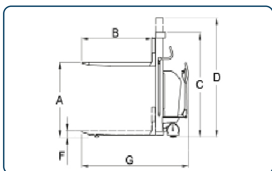
Måttskiss LF Staplare
